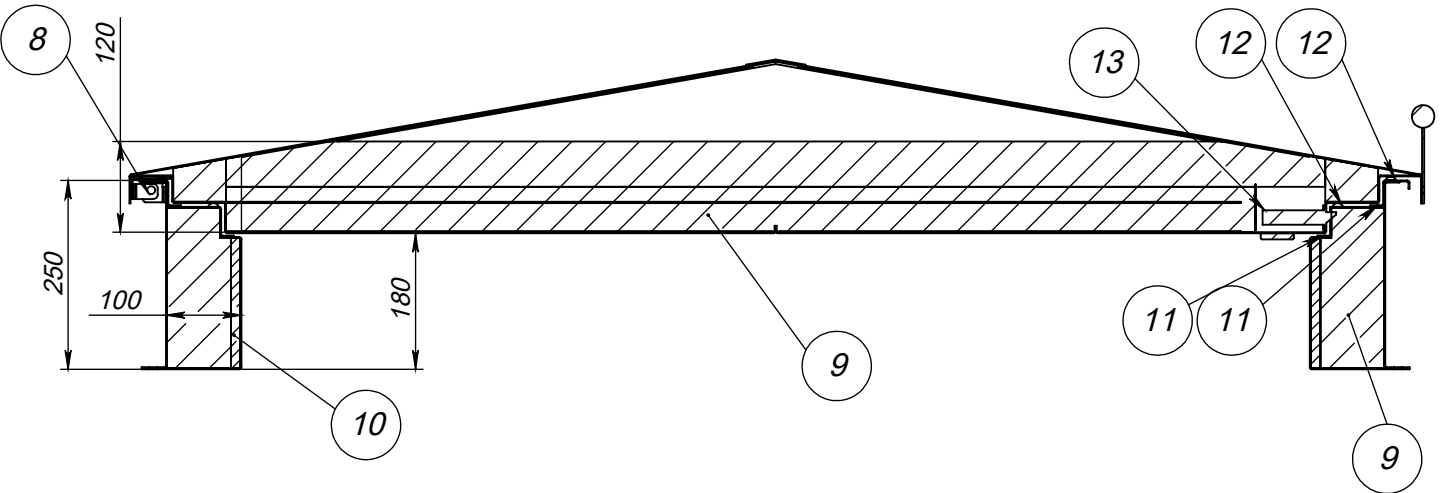
СЕЧЕНИЕ В-В МАСШТАБ 1:10
