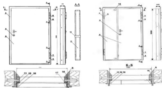
Рис. 1 Двери противопожарные металлические однопольная и двупольная
